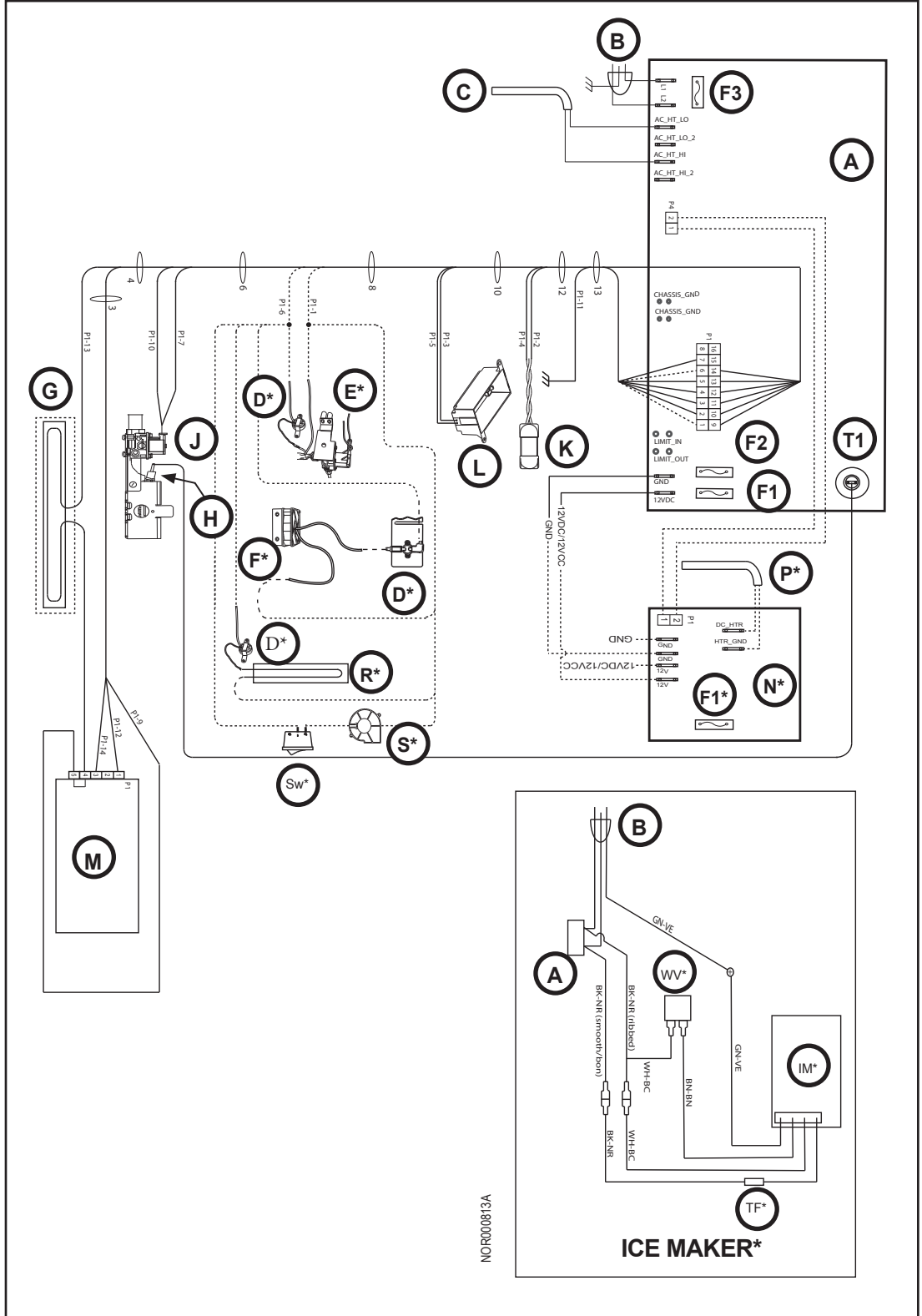
Fig. 17 - Wiring pictorial
