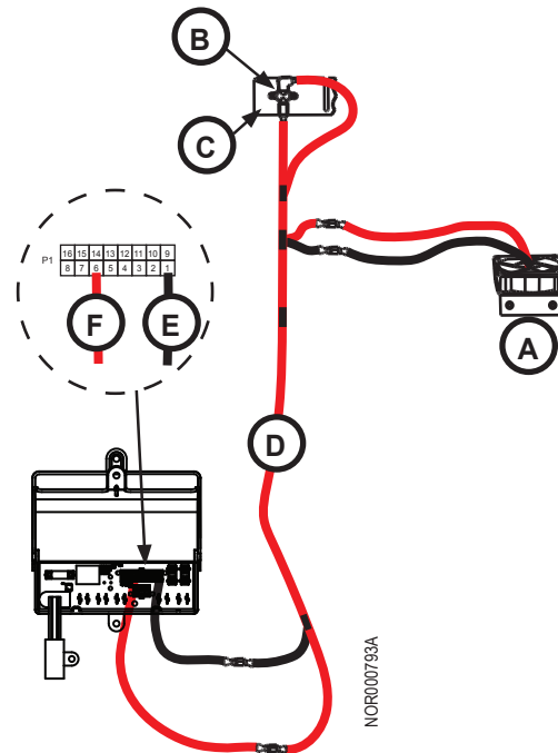
Fig. 8 - Fan wiring
