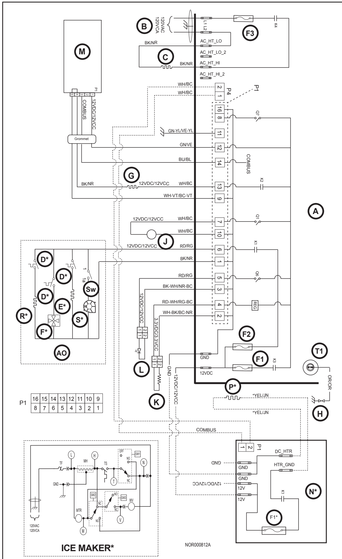
Fig. 16 - Wiring diagram
